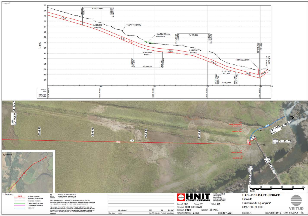
Mynd 16: Teikning af heitavatnsleiðslu 7/7. (Veitur)
