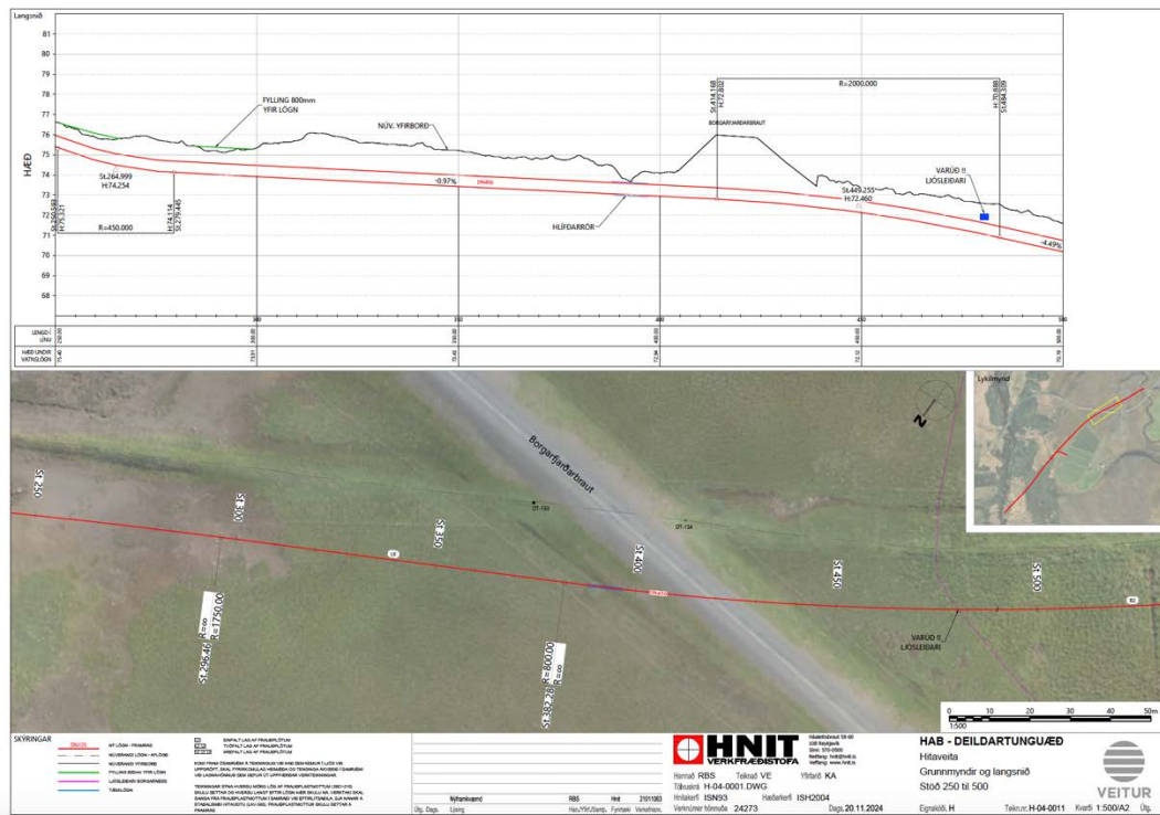
Mynd 11: Teikning af heitavatsleiðslu 2/7. (Veitur)
