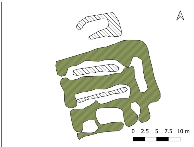
Mynd 9: Uppmæling af beitarhúsum HV-275:042.
