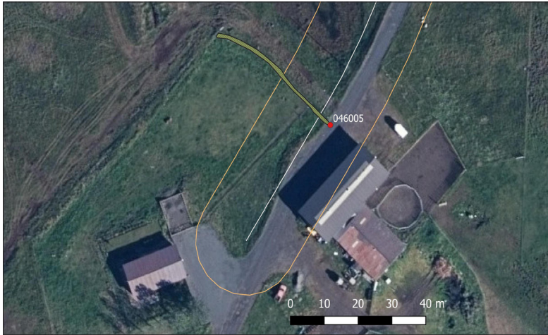
Mynd 18: Uppmæling af túngarði ÁR-046:005.
