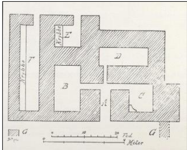
Mynd 8 - Grunnteikning af bæjarhúsunum í Kaldárseli úr bókinni Íslenskt þjóðlíf í þúsund ár eftir Daniel Bruun. A. bæjarstæði. B. baðstofa. C. eldhús. D. búr. E. hesthús með stalli. F. fjárhús með jötu. G-G kálgarðsveggir.
