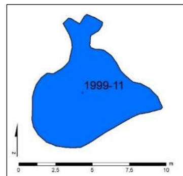
Mynd 338. Teikning af ummáli steypuleifanna (1999-11) á Lyngbergi, eftir uppmælingu.
