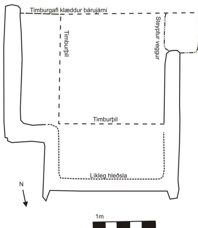
Teikning 26 Fjárhúsið í Geirakoti.
