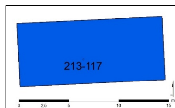
Mynd 175. Braggagrunnur (213-117), teiknað eftir uppmælingu.
