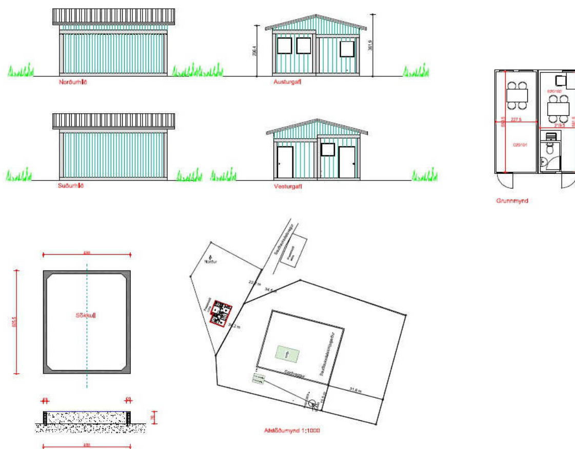
Mynd 4: Skipulagstillaga fyrir þjónustuhús við Sauðlauksdalskirkju. Tillagan gerir ráð fyrir því að útlit hússins og klæðning verði í stíl við kirkjuna. (Guðbjartur Á. Ólafsson, 2019)
