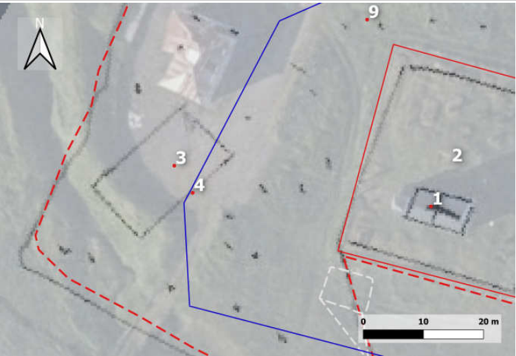
Mynd 18: Á ljósmynd frá 1939 sést torfkofi neðan við matjurtagarð (nr. 2089-3). (Teikn. ÓLA á loftmynd frá Loftmyndum ehf./túnakort frá Þjóðskjalasafni Ísl.)
