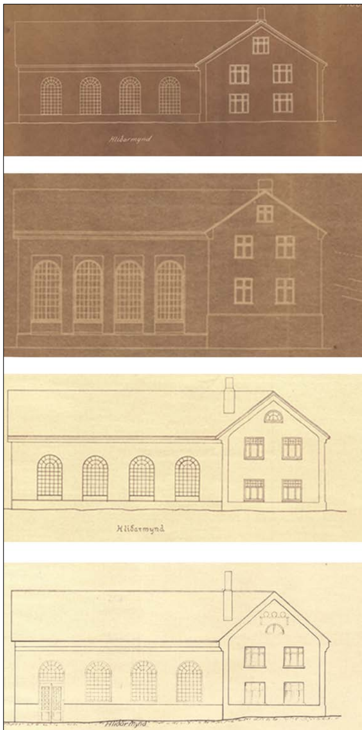
Mynd 23 Hönnunarferli rafstöðvarhússins, útlitsteikningar frá 1918, 1919, 1920 og 1921. Form og stíll hússins er með svipuðu sniði milli teikninga en staðsetning stromps, útlit glugga og staðsetning hurðar breytast milli ára. 84
