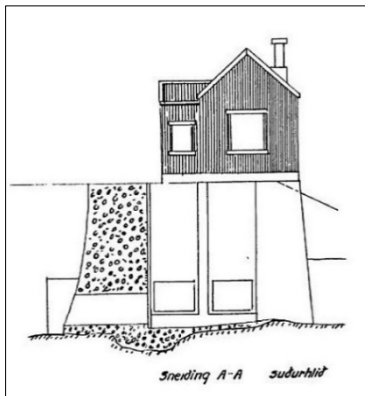
Mynd 21 Teikning af suðurgafli stífluhúss (áður eitt af veiðihúsunum) eftir flutning að Árbæjarstíflu árið 1930. 78
