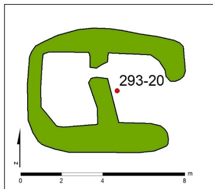
Mynd 32. Teikning af tóft 293-20 eftir uppmælingu.
