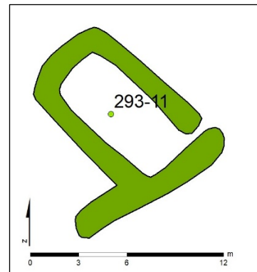
Mynd 27. Rúst (293-11), teiknuð eftir uppmælingu.
