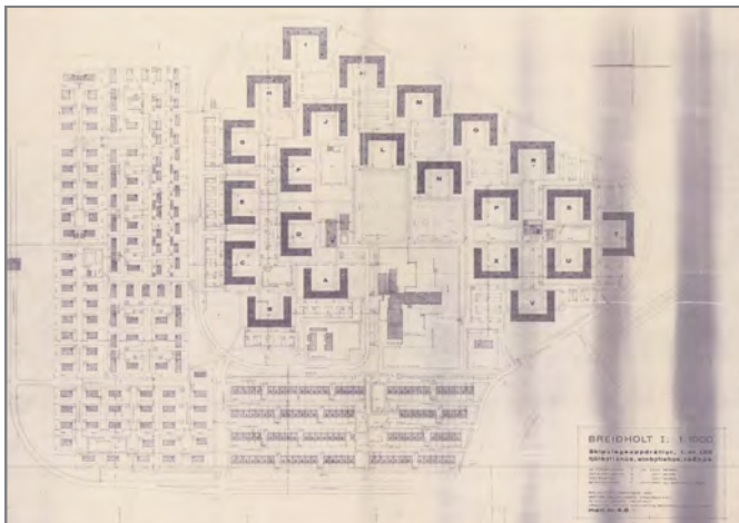
Breiðholt I, Bakkar og Stekkir. Skipulagsuppráttur frá 1966 eftir Reyni Vilhjálmsson og Stefán Jónsson arkitekta.
