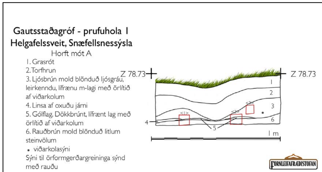
Mynd 54. Prufuhola I í rúst 3. Sniðteikning. Á myndinni sést einnig hvar sýni voru tekin til örformgerðargreininga.
