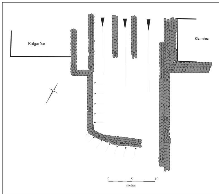
Mynd 32. Uppdráttur af bryggjunni Steingerði 018
