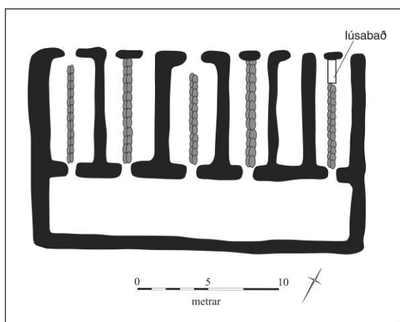
Mynd 12. Uppdráttur af fjárhúsum 005
