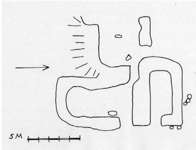
Mynd 14. Flatarteikning, tóft nr. 11. Teikn. K.G. sept. 2000
