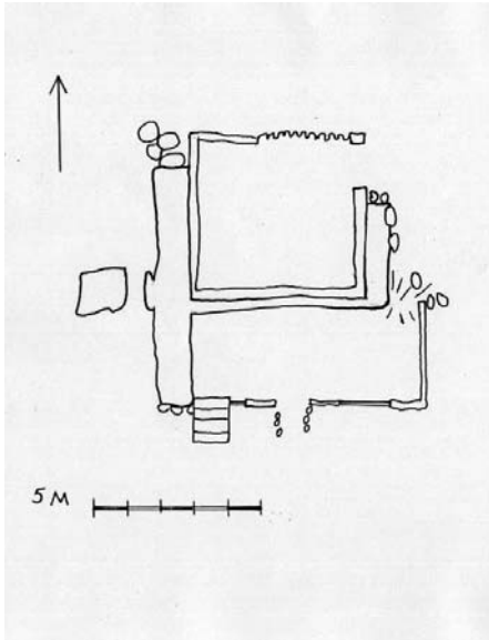
Mynd 31. Flatarteiking, tóft. Teikn. K.G. júlí 2000
